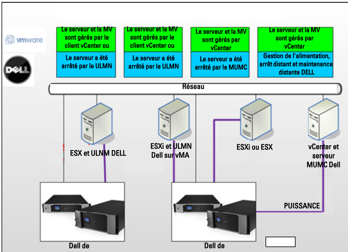
Schéma 82. ULMN Dell Configurations du schéma VMware
