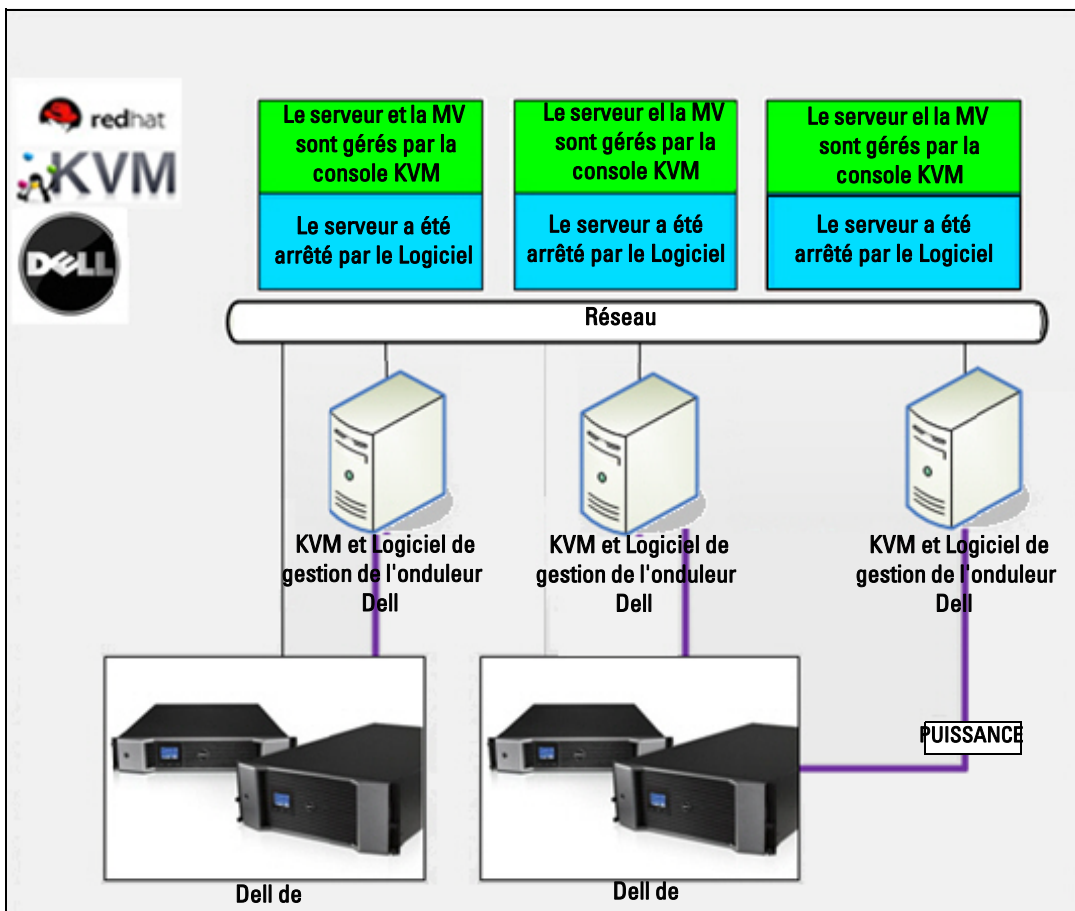
Schéma 96. Solutions ULNM Dell pour Red Hat KVM ou Open-source KVM
